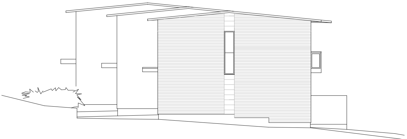
JULKISIVU LUOTEESEEN
